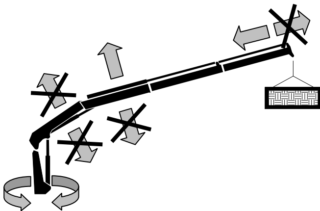
2° braccio sopra l'orizzontale 2 nd boom over the horizontal line 2. Ausleger über der Horizontale
