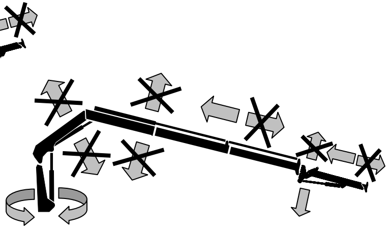
2° braccio e braccio jib sotto l'orizzontale 2 nd boom and jib boom under the horizontal line 2. Ausleger und Jib-Ausleger unter der Horizontale
