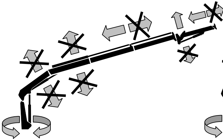
2° braccio e braccio sopra l'orizzontale 2 nd boom and jib boom over the horizontal line 2. Ausleger und Jib-Ausleger über der Horizontale
