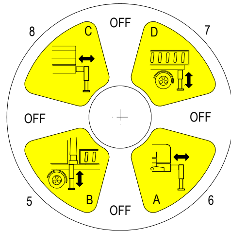
Lato opposto distributore Opposite control valve side Gegenseite des Steuerventil
