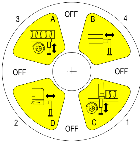
Lato distributore Control valve side Seite des Steuerventil
