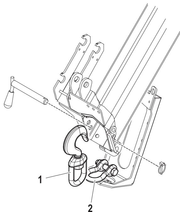
posizionamento 4S placement 4S - E4
