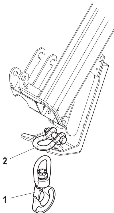
posizionamento 2S placement 2S - E2
